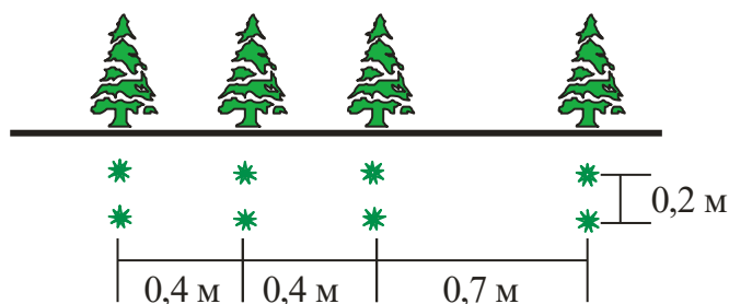
Рис. 4. Схема уплотненной школы
